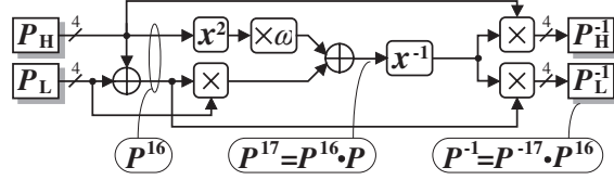
Fig. 4. \text{GF}((2^4)^2) inverter
